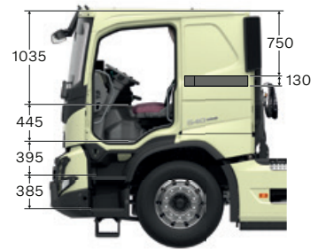
NIEDRIGES LANGES FAHRERHAUS
